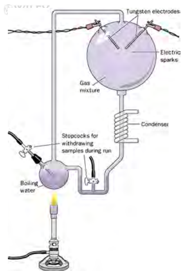
ユリーとミラーの実験装置: 原始地球上での有機化合物をまねる実験装置 (1953年)
