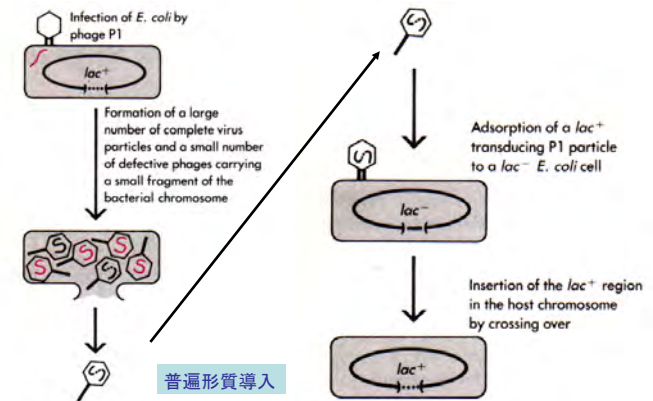
P1 トランスダクション
