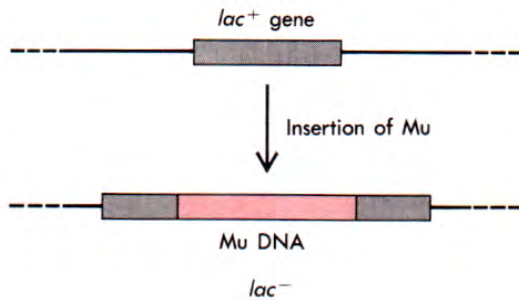
Muは入ファージと異なり、挿入が起こる場所はランダムである
