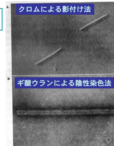
TMV粒子の 電子顕微鏡写真
